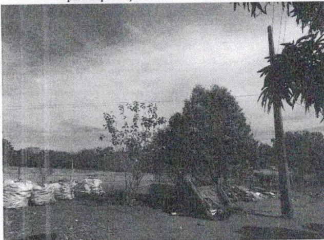
Foto 3 - Final de Rede de BT e poste com IP - Trecho complementar para implantação de IP
