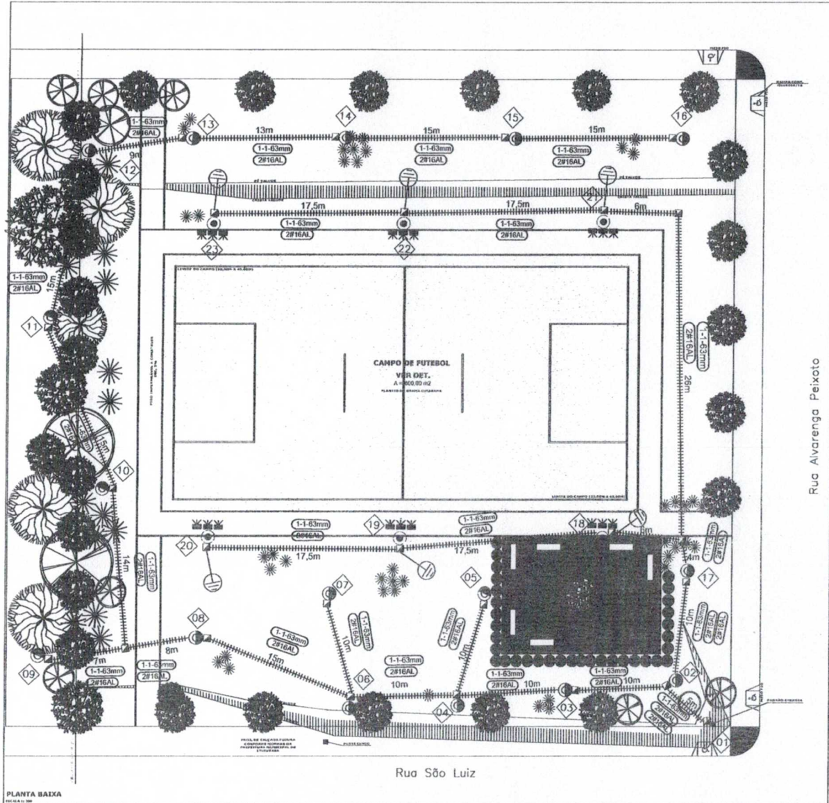
PLANTA BAIXA
